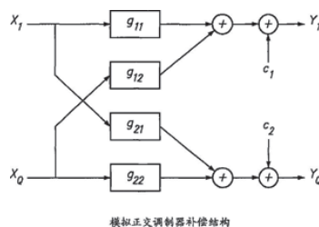
模數正交調制器補償結構
