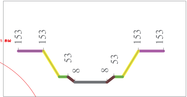
橫切面BB' Secção Longitudinal BB'
