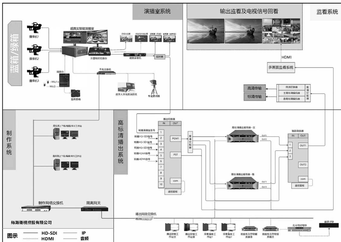
Anexo: Fluxograma do Sistema de Produção e Transmissão Televisiva
