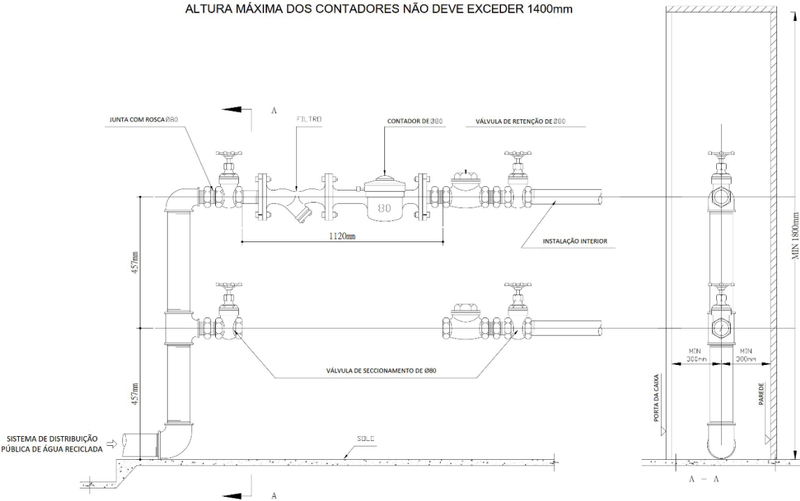
Figura 9 Esquema para colocação de contador de Ø80
