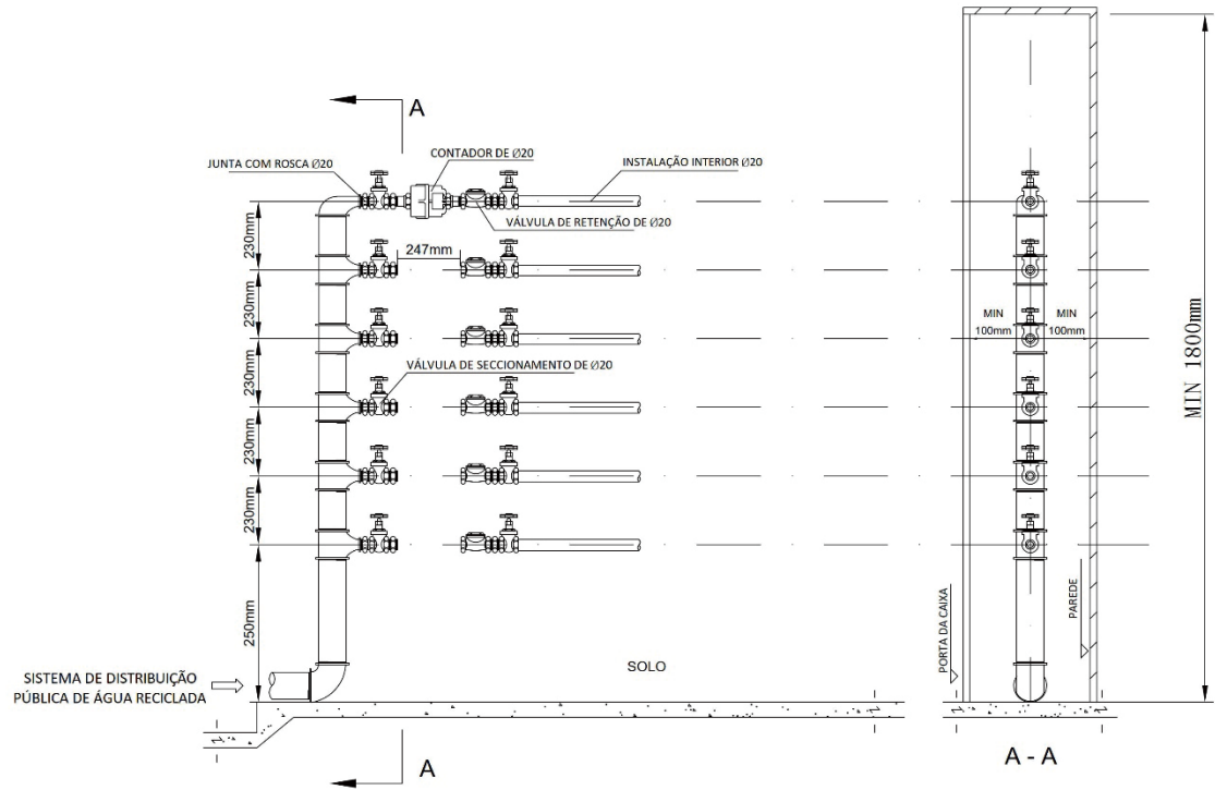
Figura 6 Esquema para colocação de contador de Ø25
