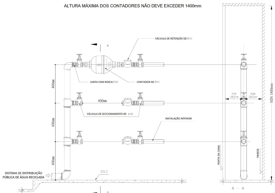
Figura 7 Esquema para colocação de contador de Ø40
