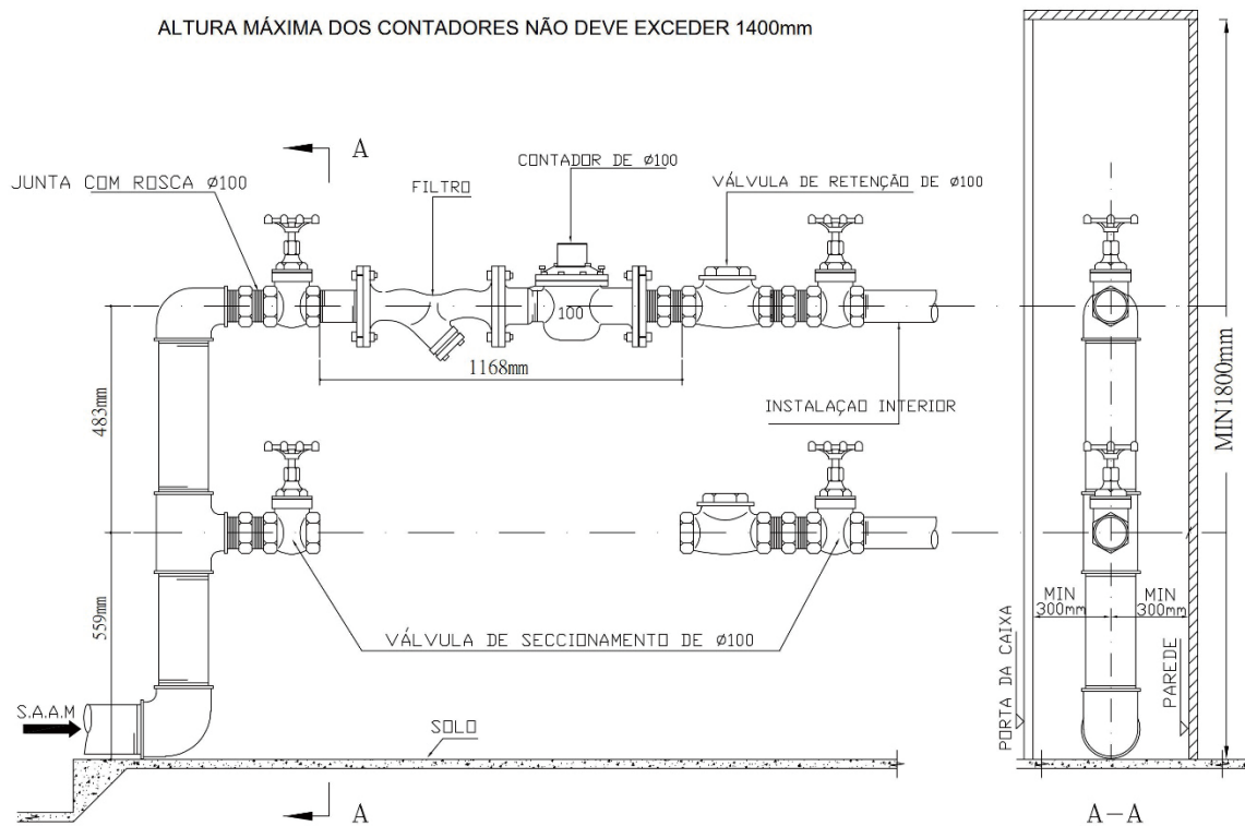
Figura 11 Esquema para colocação de contador de Ø100
