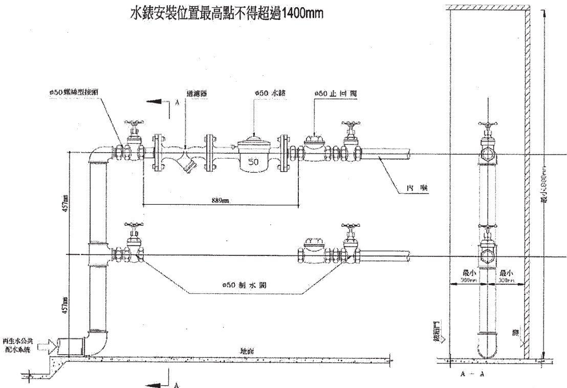
圖八 Ø50水錶安裝的圖解
