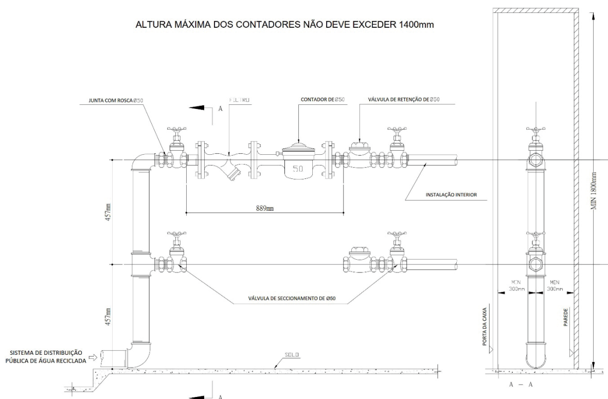
Figura 8 Esquema para colocação de contador de Ø50
