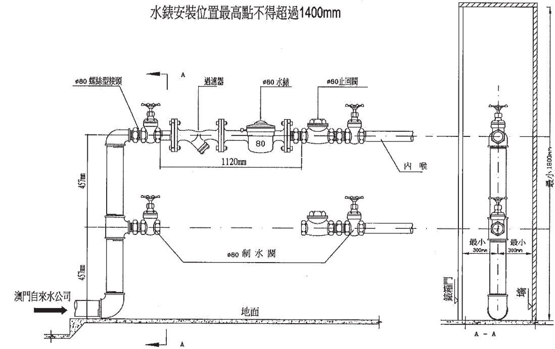
圖十 Ø80水錶安裝的圖解
