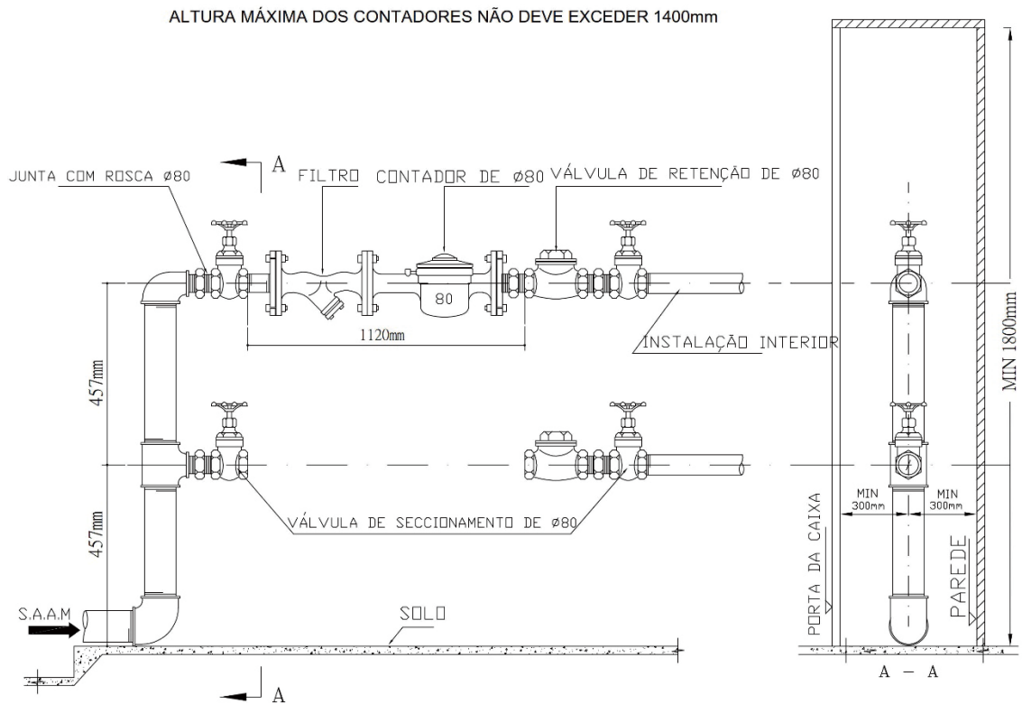
Figura 10 Esquema para colocação de contador de Ø80
