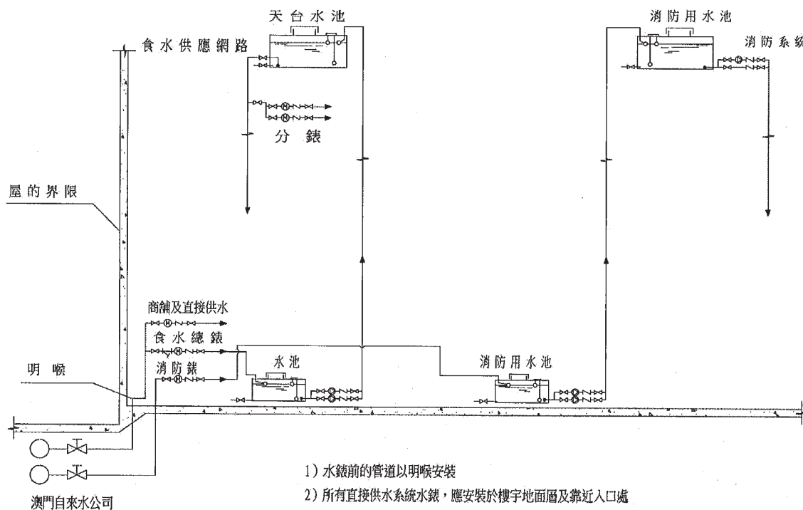
圖二 間接供水系統
