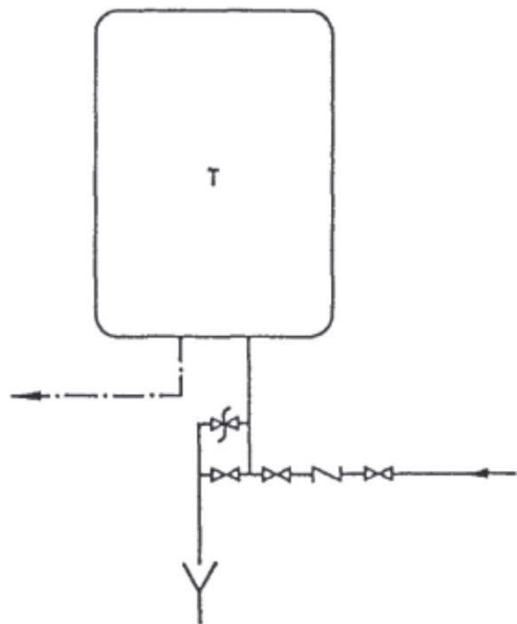
附件十六 (第一百八十八條第五款所指者) 儲水式熱水器的接連類型圖解
