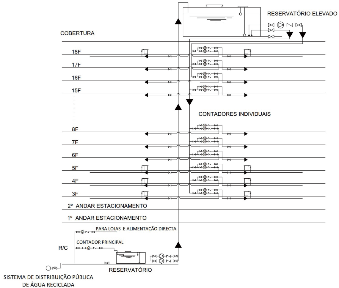
Figura 2 Sistema indirecto de abastecimento de água
