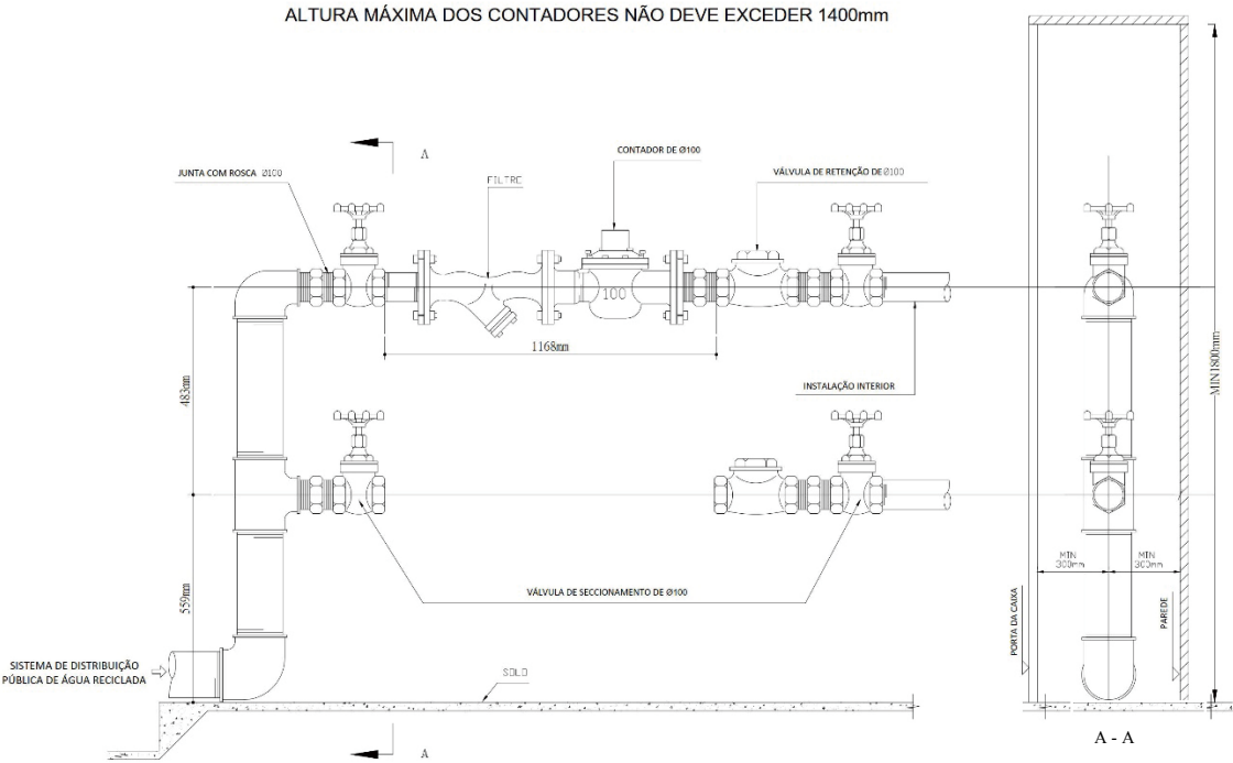
Figura 10 Esquema para colocação de contador de Ø100
