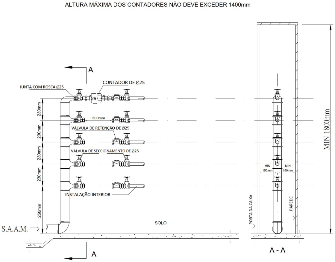
Figura 7 Esquema para colocação de contador de Ø25
