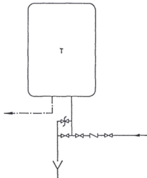
ANEXO XVI (a que se refere o n.º 5 do artigo 188.º) Esquemas tipo de ligação de termoacumuladores
