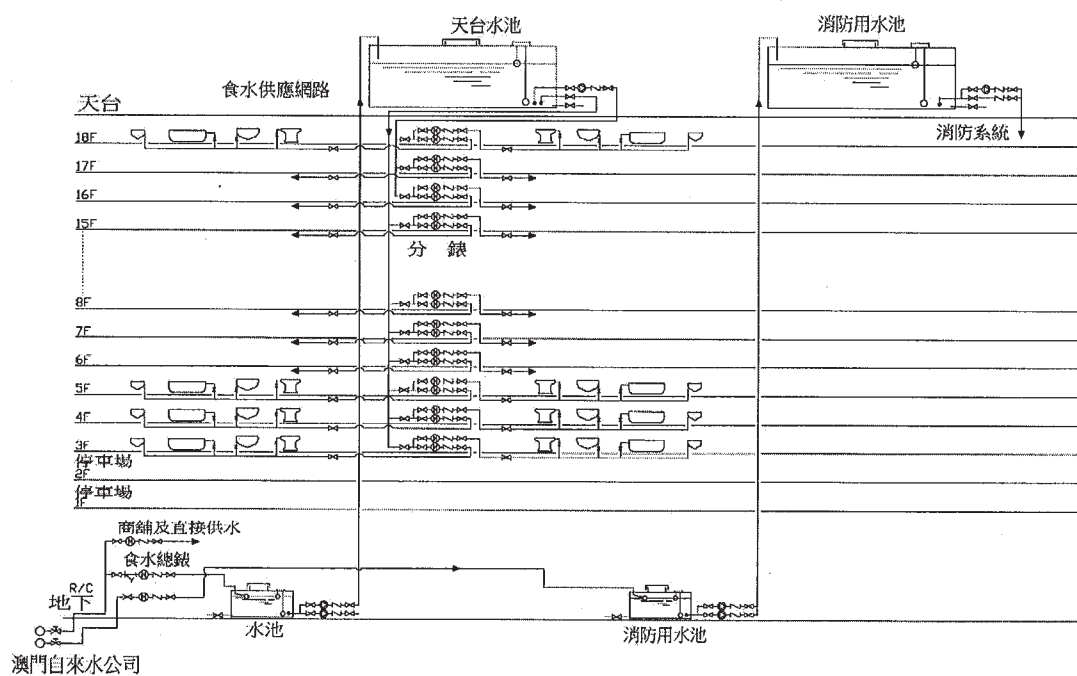
圖三 間接供水系統
