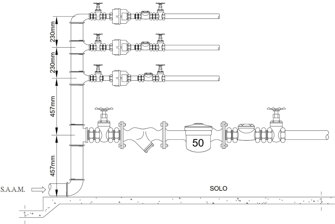
Figura 5 Esquema para colocação de contador de Ø15
