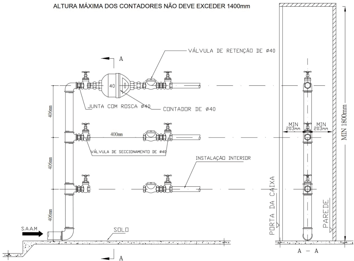
Figura 8 Esquema para colocação de contador de Ø40
