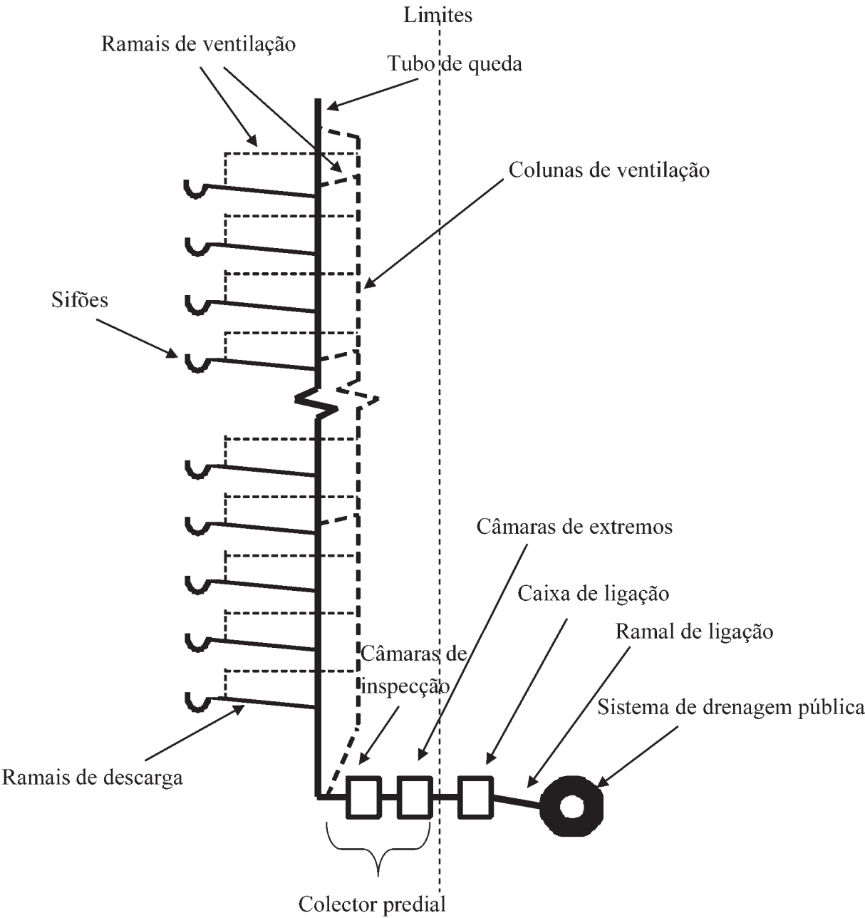
Diagrama esquemático do sistema predial de drenagem de águas residuais
