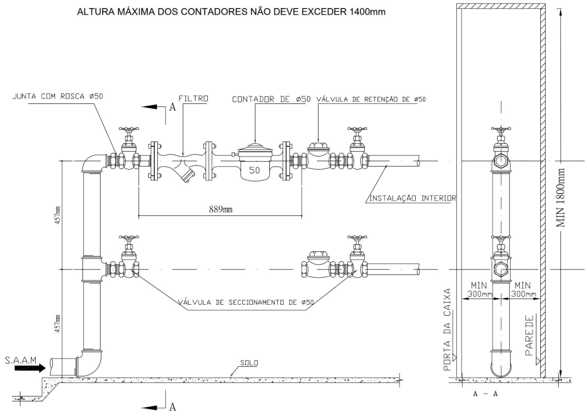
Figura 9 Esquema para colocação de contador de Ø50
