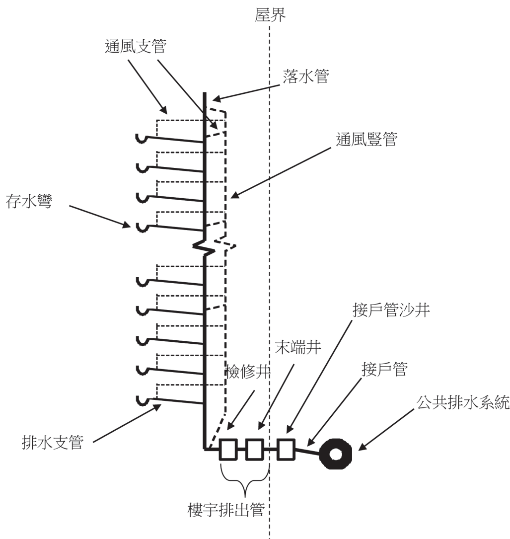
樓宇廢水排放系統示意圖
