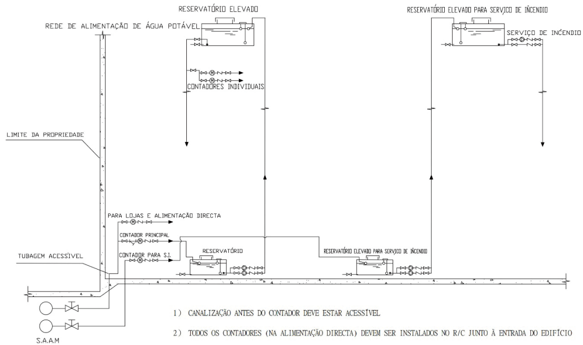
Figura 2 Sistema indirecto de abastecimento de água
