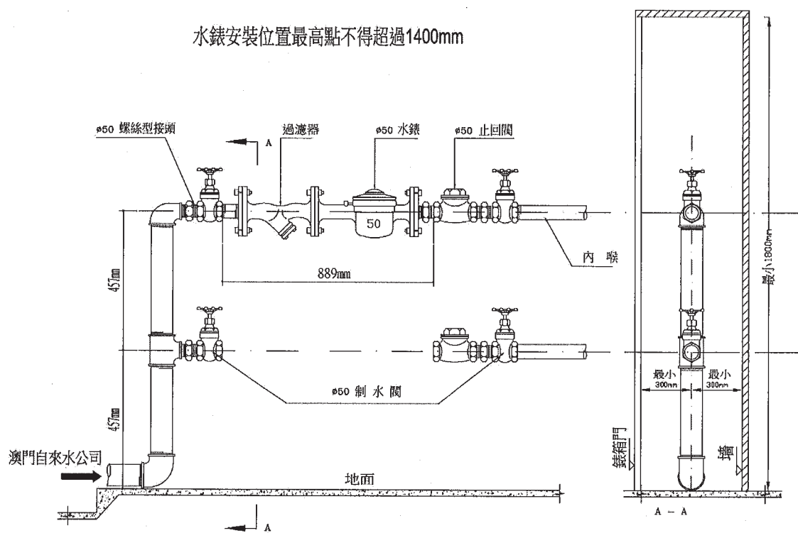
圖九 Ø50水錶安裝的圖解
