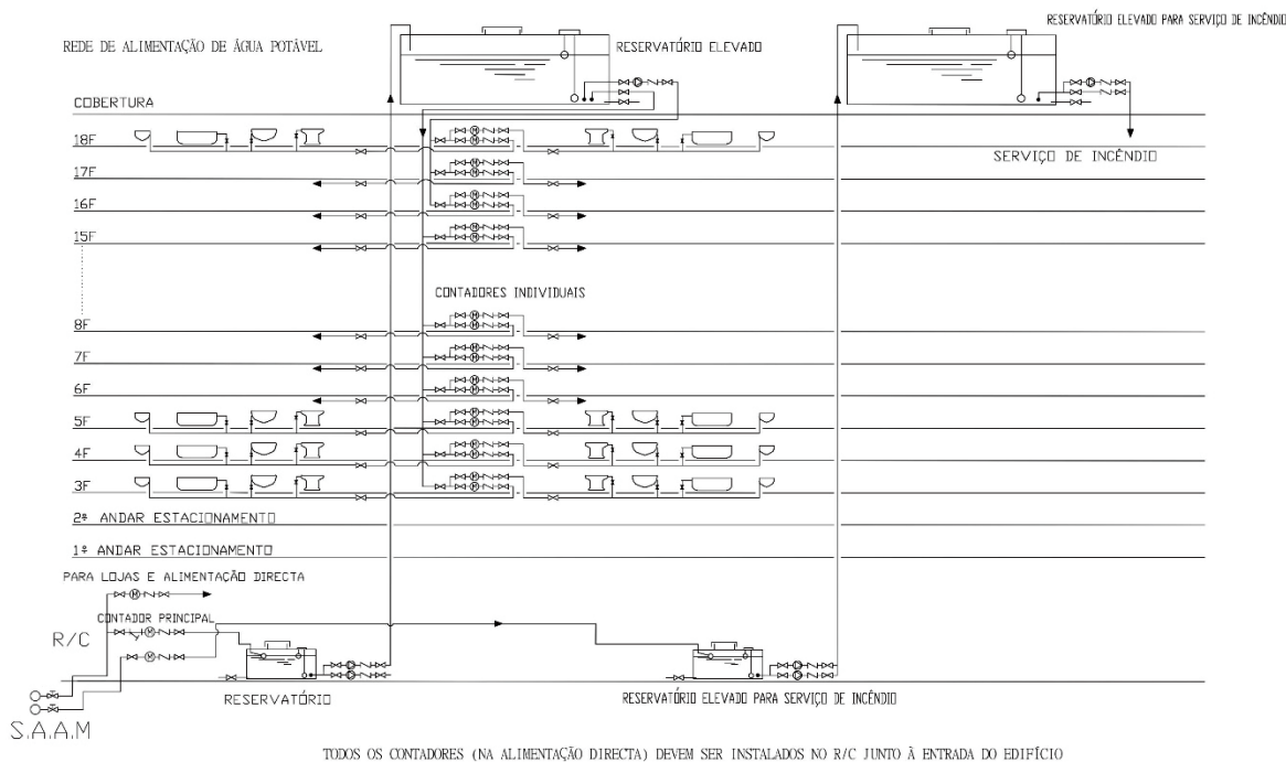
Figura 3 Sistema indirecto de abastecimento de água
