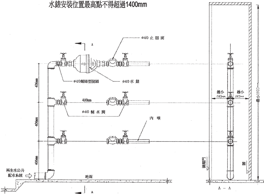
圖七 Ø40水錶安裝的圖解
