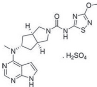
式 (I)
