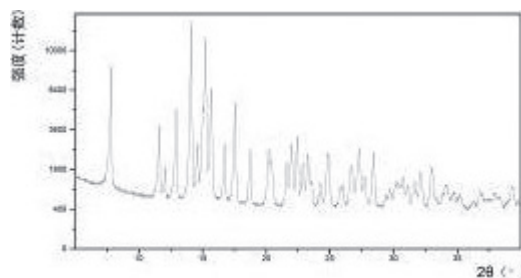
HPC 后進行 SD 之後的糠酸莫米松一水合物的 XRPD 衍射圖
