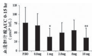
在研究NB4-02-06-003中，LUM001降低血清膽汁酸AUC 0-15 hr (在第14天測定；與安慰劑相比，*p < 0.05, **p < 0.01)
